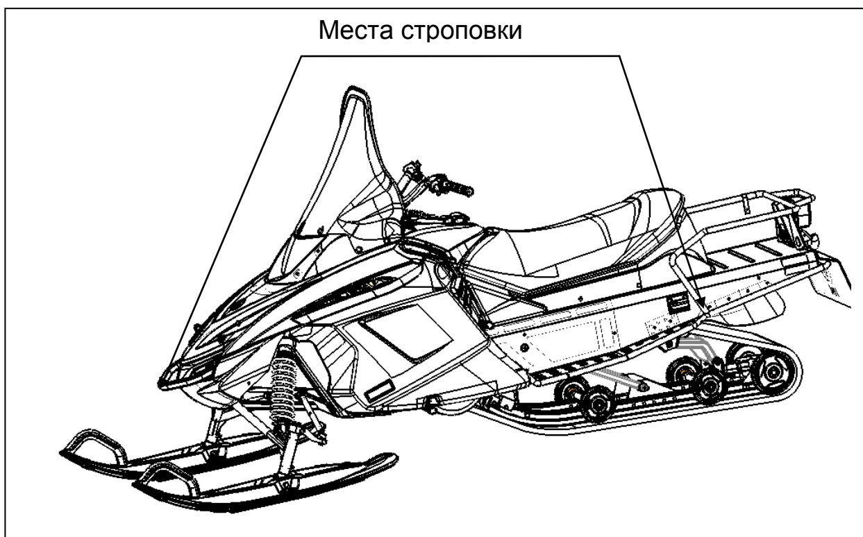
Рисунок 13 – Строповка снегохода
