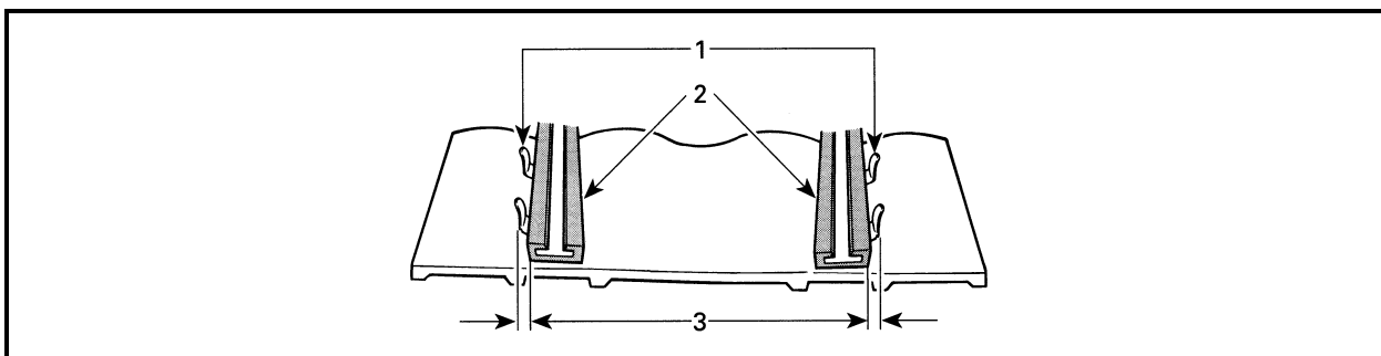
Рисунок 21 – Проверка симметричности положения гусеницы
