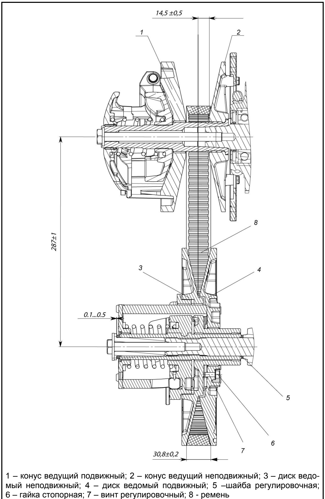
Рисунок 17 – Регулировка вариатора
