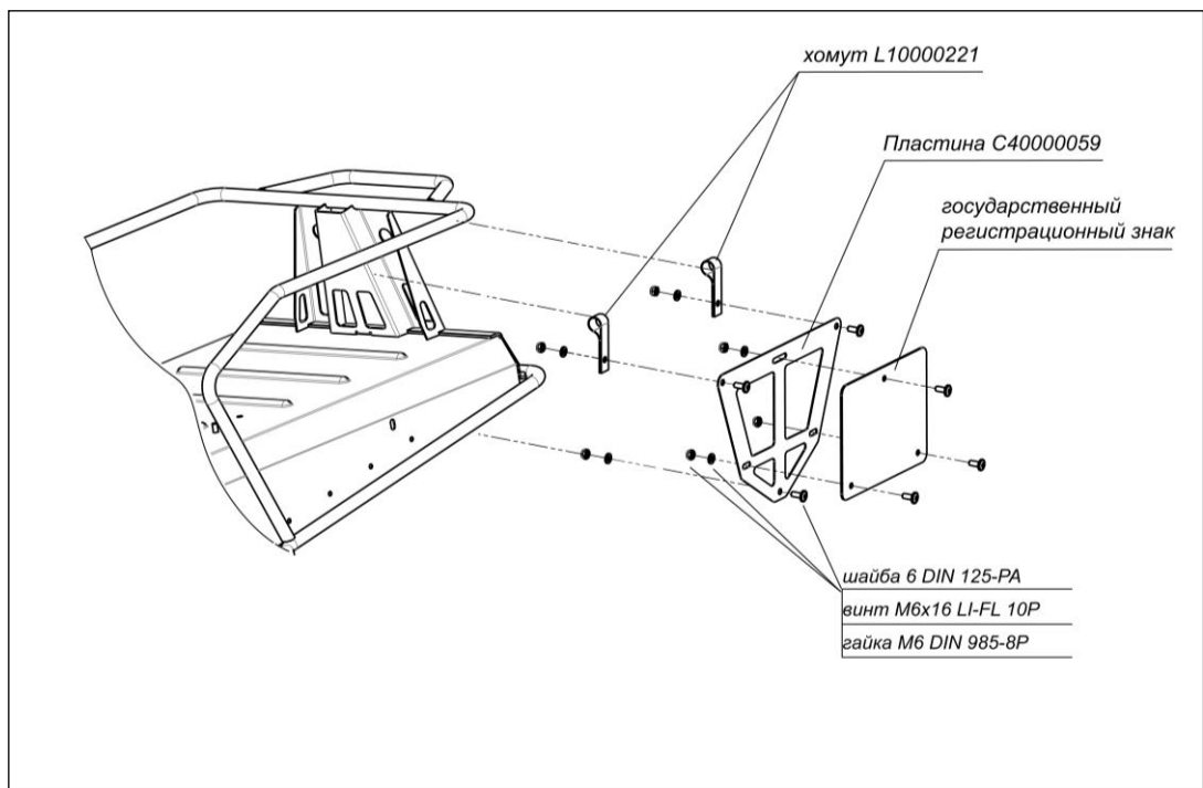
Рисунок 3 - Крепление государственного регистрационного знака
